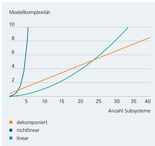
Lineare Anstieg der Modellkomplexität mit der Anzahl der Komponenten durch Dekomposition von Parametertensoren multilinear Modelle 1
